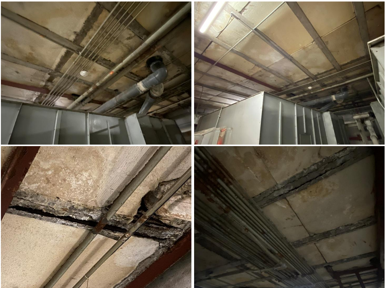
“VIGUETAS EN SISTEMA DE LOSA DE EQUIPOS, SOBRE CUARTO DE COMPRESORES”.
